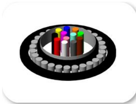
GPMXTC33 GPMXTCY33 Item Code:STFFC-GPMXTC(Y)33
